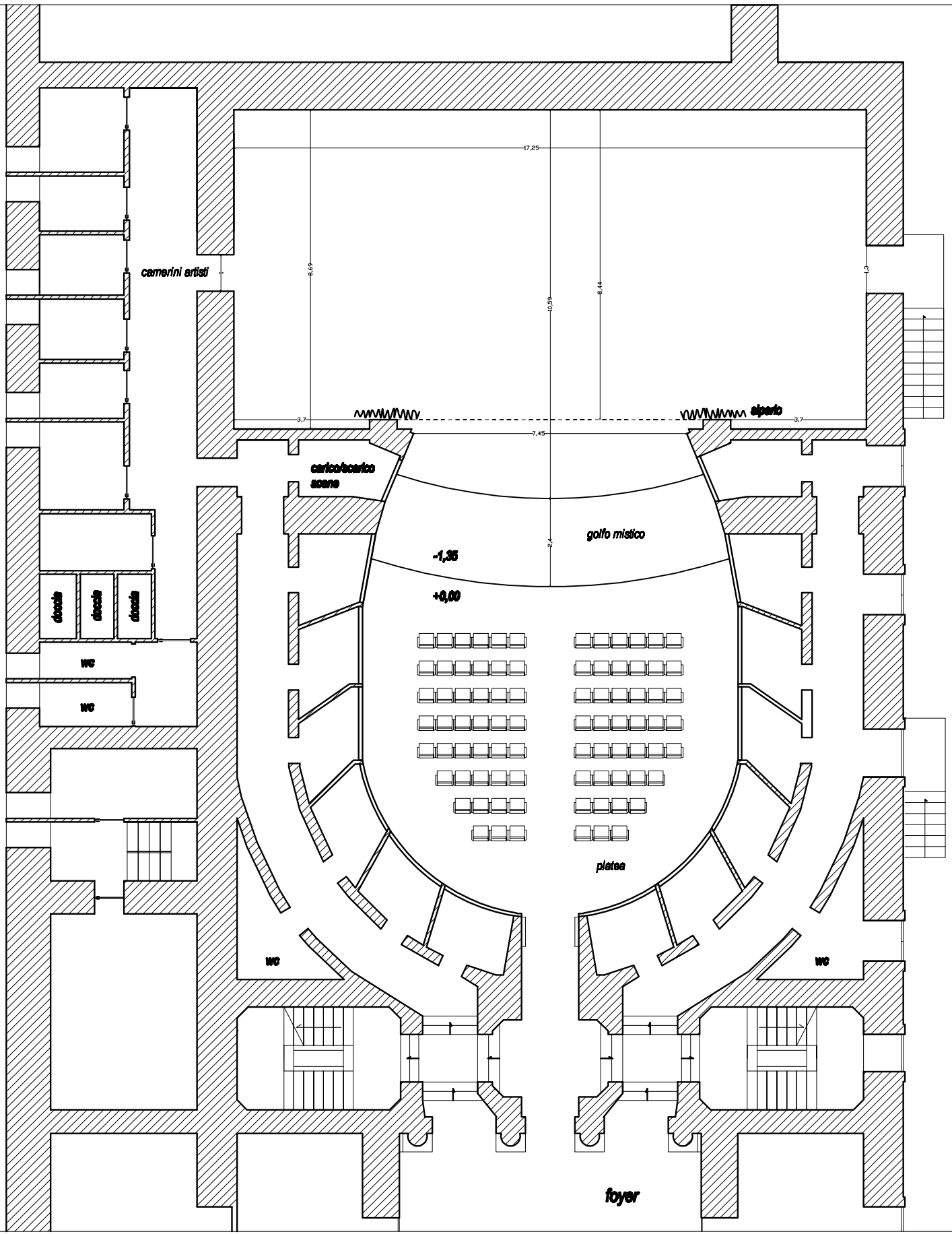
Teatro Vitt. Emanuele di Noto Pianta scala 1:100 disegno di Peppe Bonfiglio
